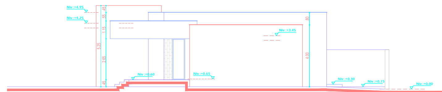
Facade Sud-Ouest
