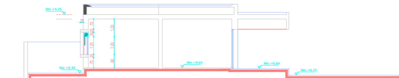
COUPE C-C
